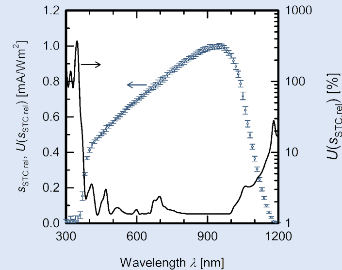
Kalibrierte Messung der spektralen Bestrahlungsstärkeempfindlichkeit s_{STC,rel} eines Strahlungssensors und der zugehörigen Messunsicherheit U
