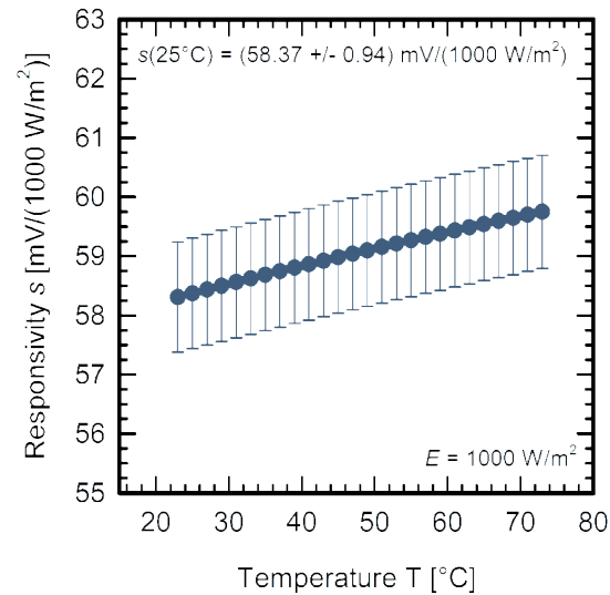
Kalibrierte Messung der Bestrahlungsstärkeempfindlichkeit s eines Strahlungssensors als Funktion der Temperatur T
